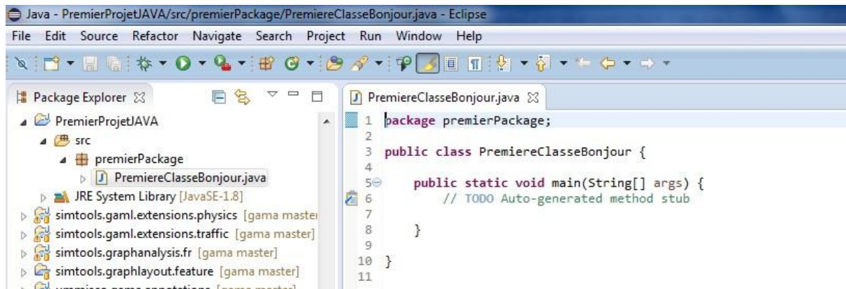
FIGURE 2.9 : CLASSE CREE
