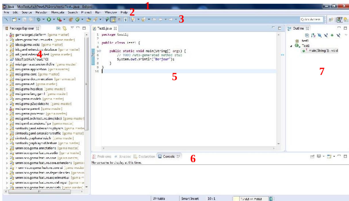
FIGURE 1.2 : WORKBENCH D'ECLIPSE
